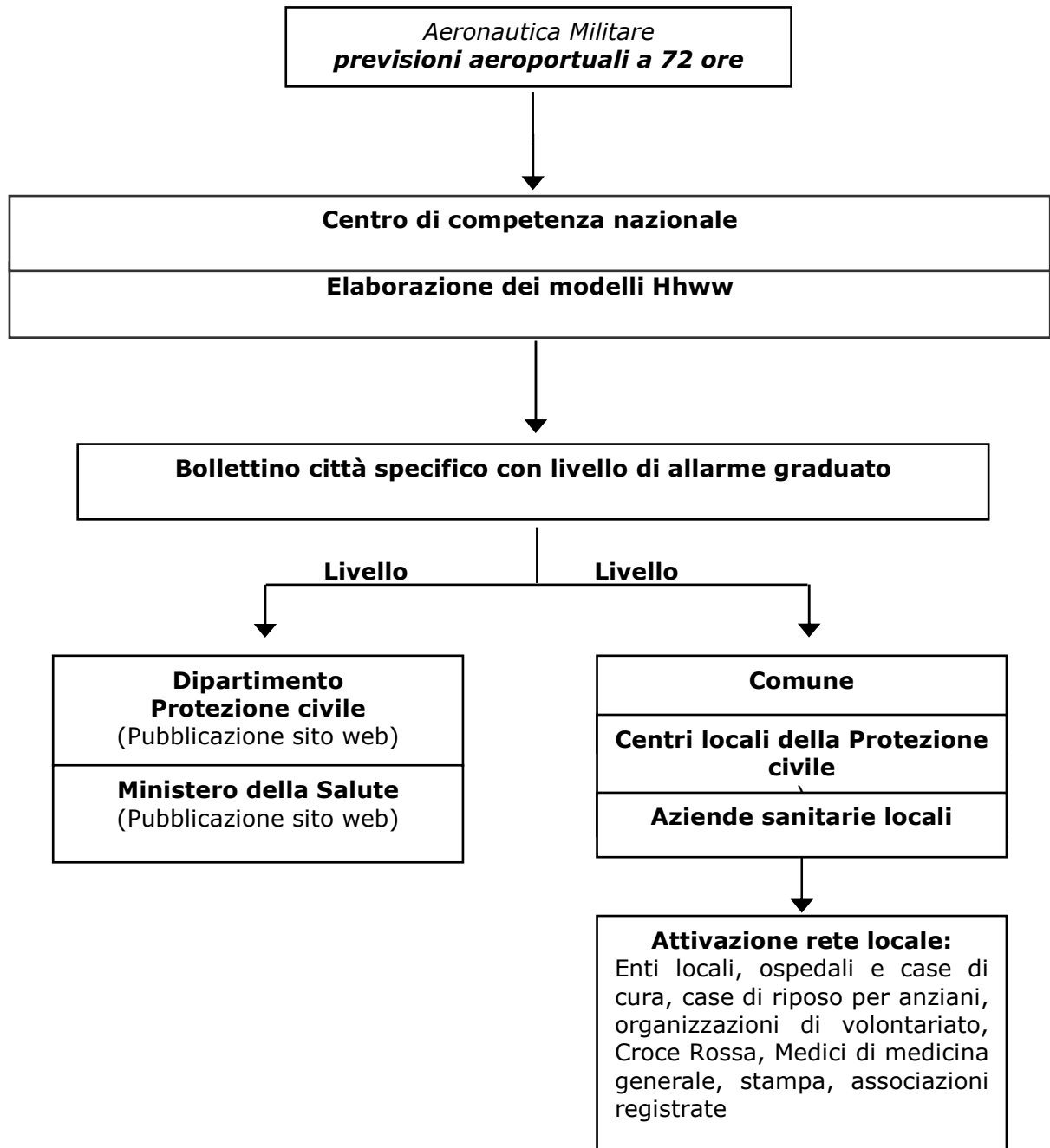
Figura 2. Schema di flusso della rete informativa per la prevenzione degli effetti del caldo sulla salute
